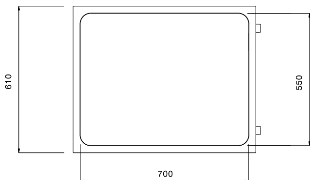
Boven aanzicht
